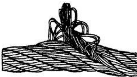
Рисунок 11. Выдавливание сердечника.
