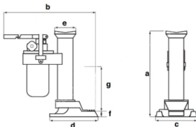
Рисунок 1. Размеры домкрата
