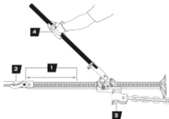
Рисунок 8. Вытягивание.
