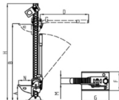
Рисунок 1. Размеры домкрата.
