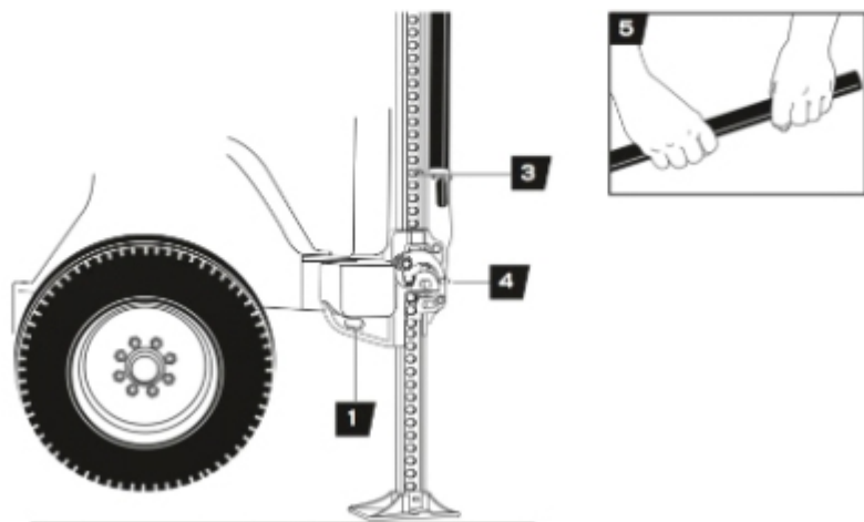
Рисунок 6. Опускание груза.
