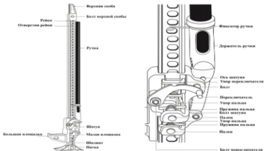
Рисунок 2. Устройство домкрата.
