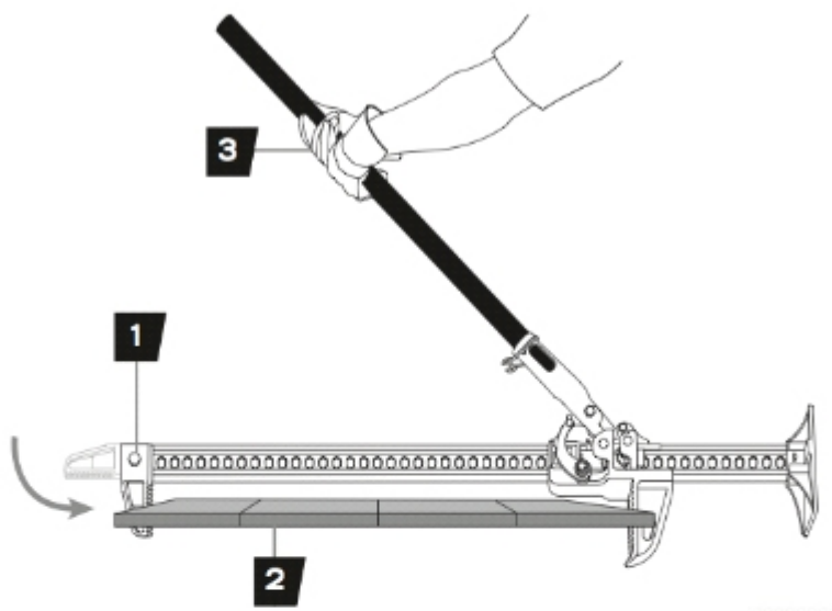
Рисунок 7. Сжатие.
